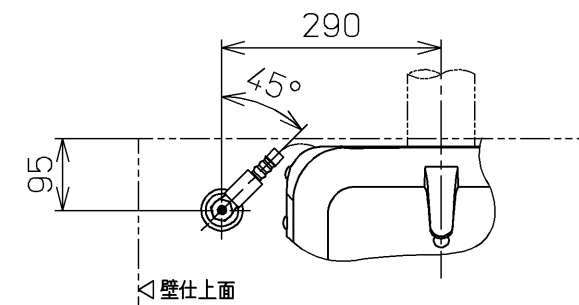
平面图
