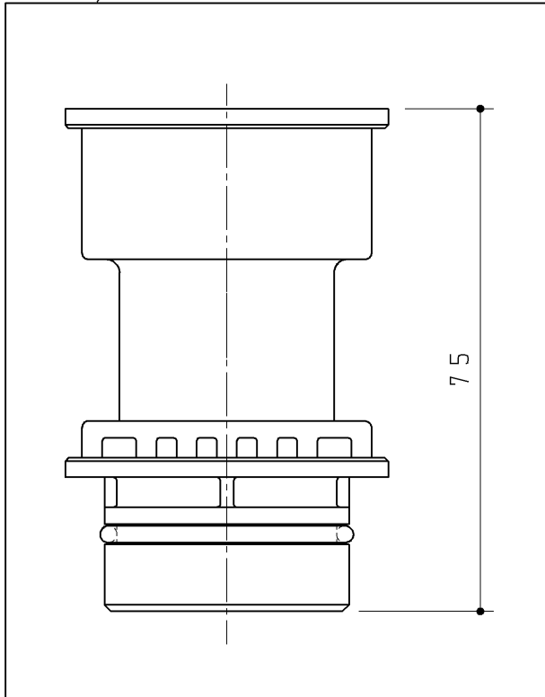
手洗排水横引管（1200）
