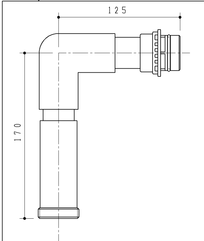
手洗排水縦管（ショート）
