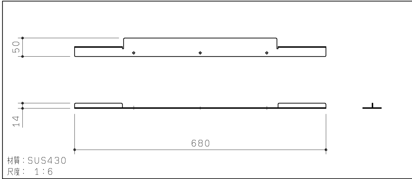
底板支持材
