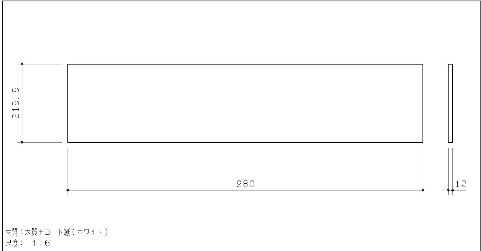
収納底板
