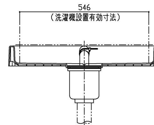
断面B-B
