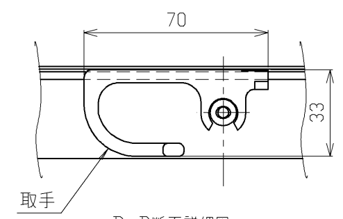
B-B断面詳細図 (1:2)
