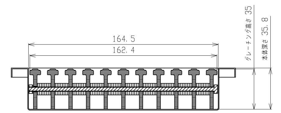
A-A断面詳細図 (1:2)
