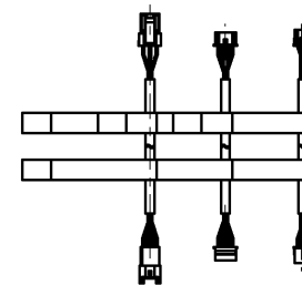
付属コード（３本、１：５）
