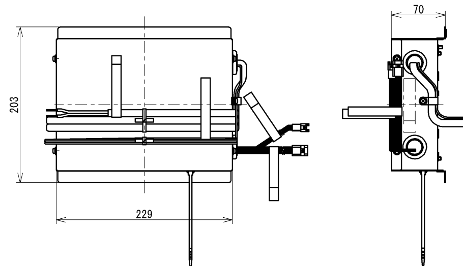
電源ボックス（１：５）
