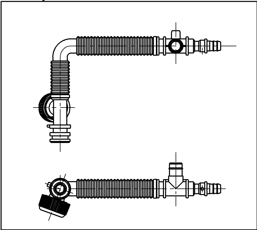
ボールタップ変更ユニット(8L用)
