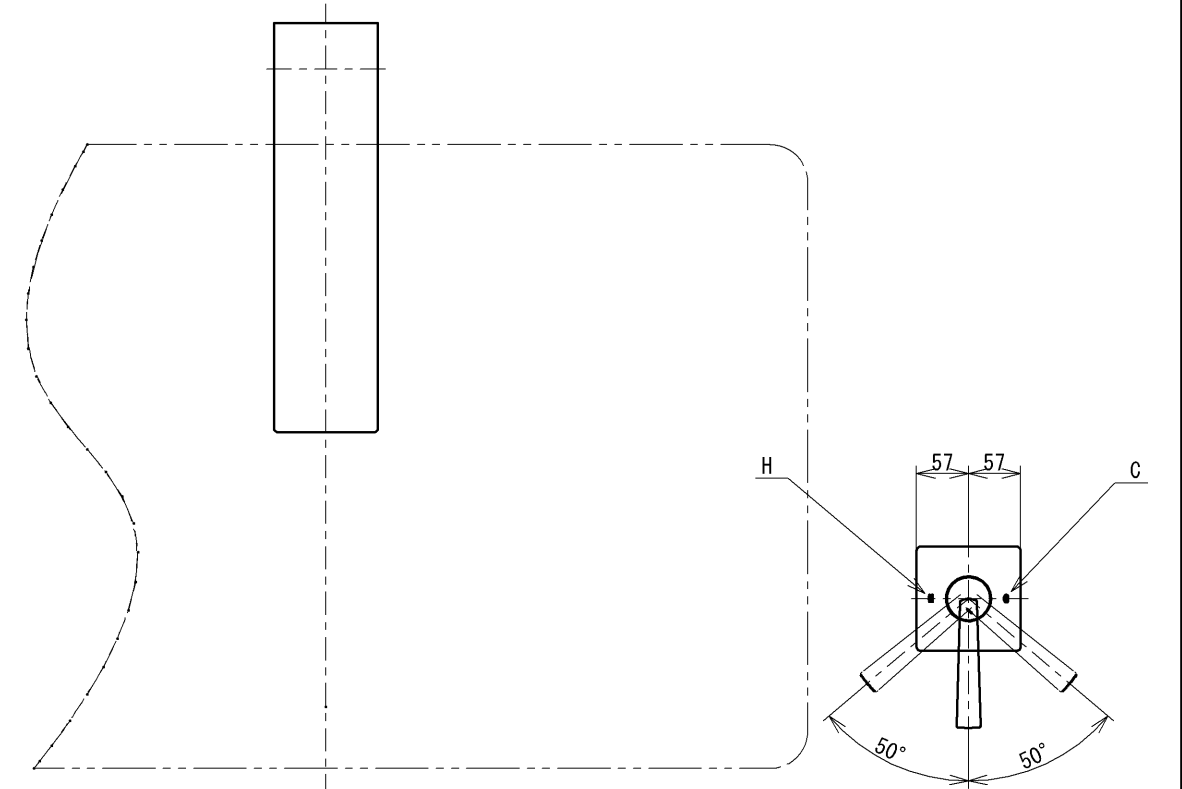
矢視図 P
