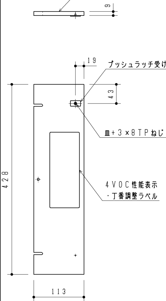
カウンター下扉裏面材
