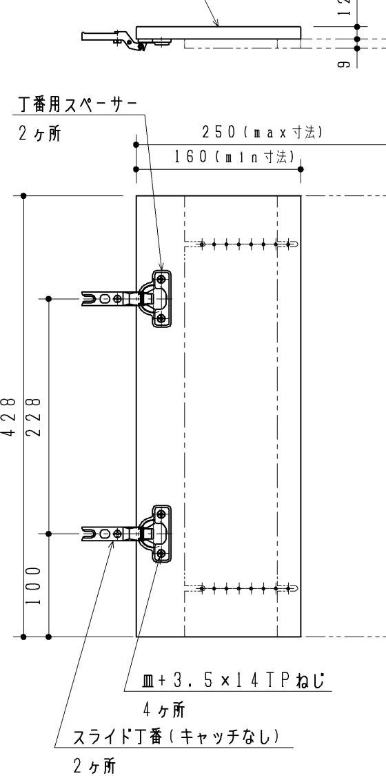
カウンター下扉表面材
