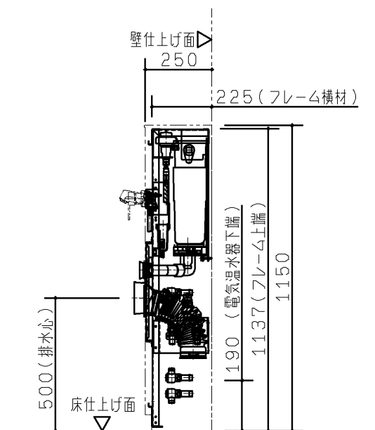
R 視図
