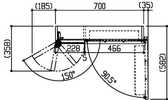
L0125L 軌跡図
