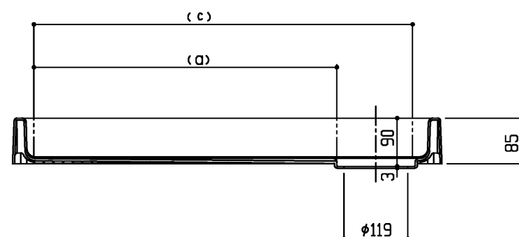
断面A-A
