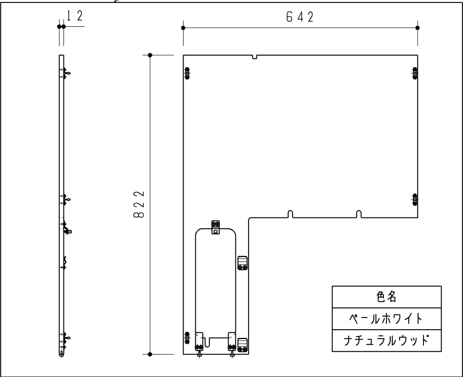
化粧側板R（奥行大）
