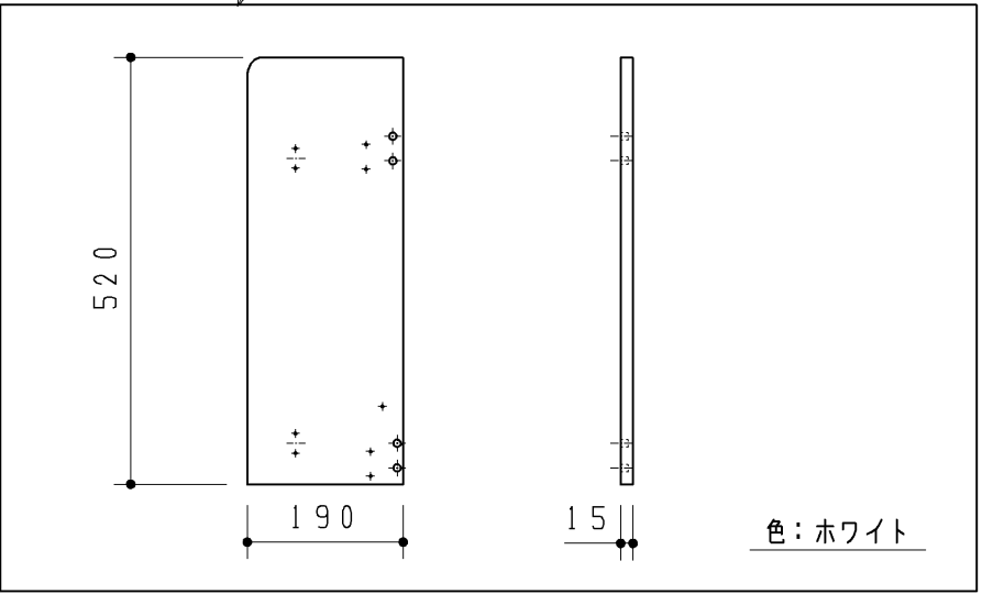
化粧側板R（奥行小）
