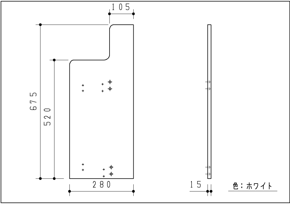
化粧側板R（奥行大）
