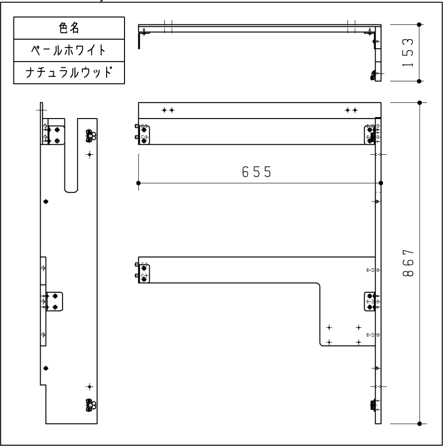
化粧側板R（奥行小）
