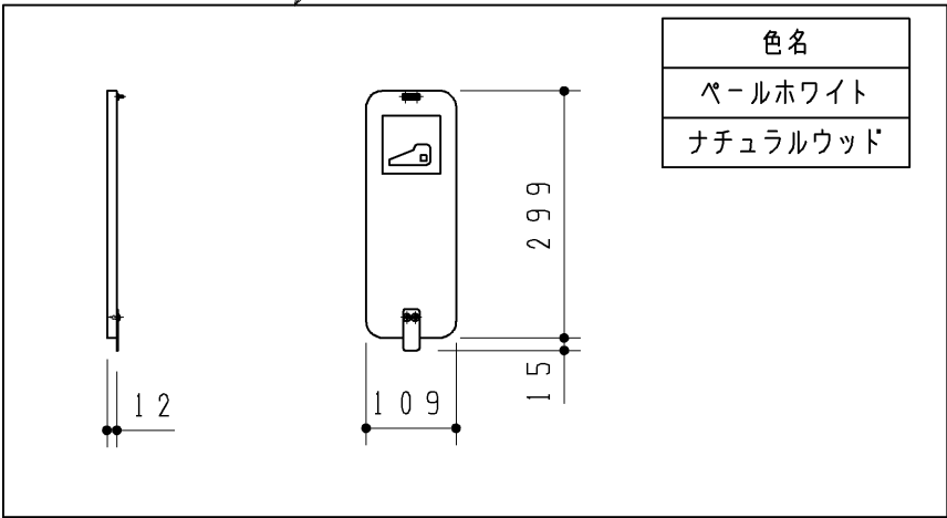
塞ぎパネルセットR
