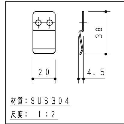
取付材 1ヶ
