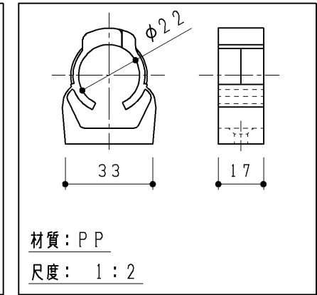
取付材 1ヶ
