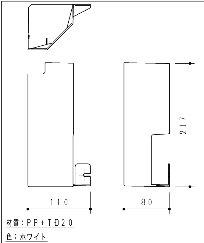
カバー（配管）
