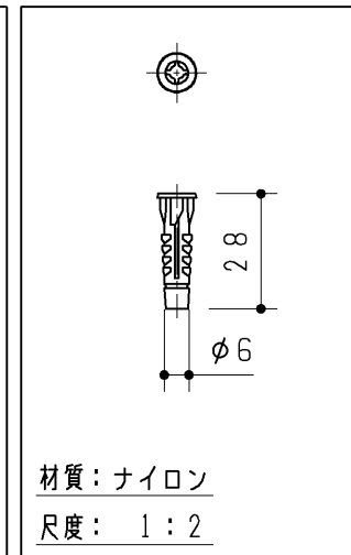
取付材 1ヶ
