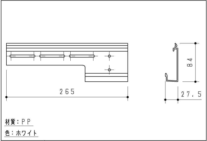
取付材
