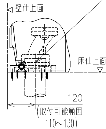
排水芯120mmの場合
