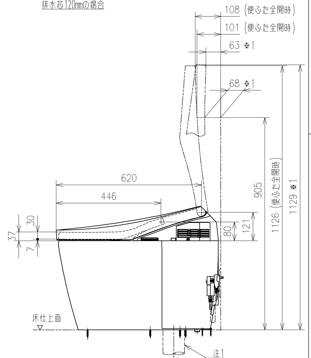
排水芯120mmの場合
