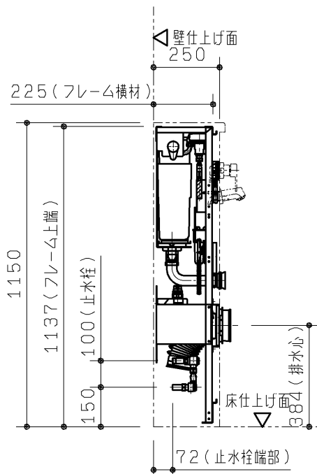
尺視圖
