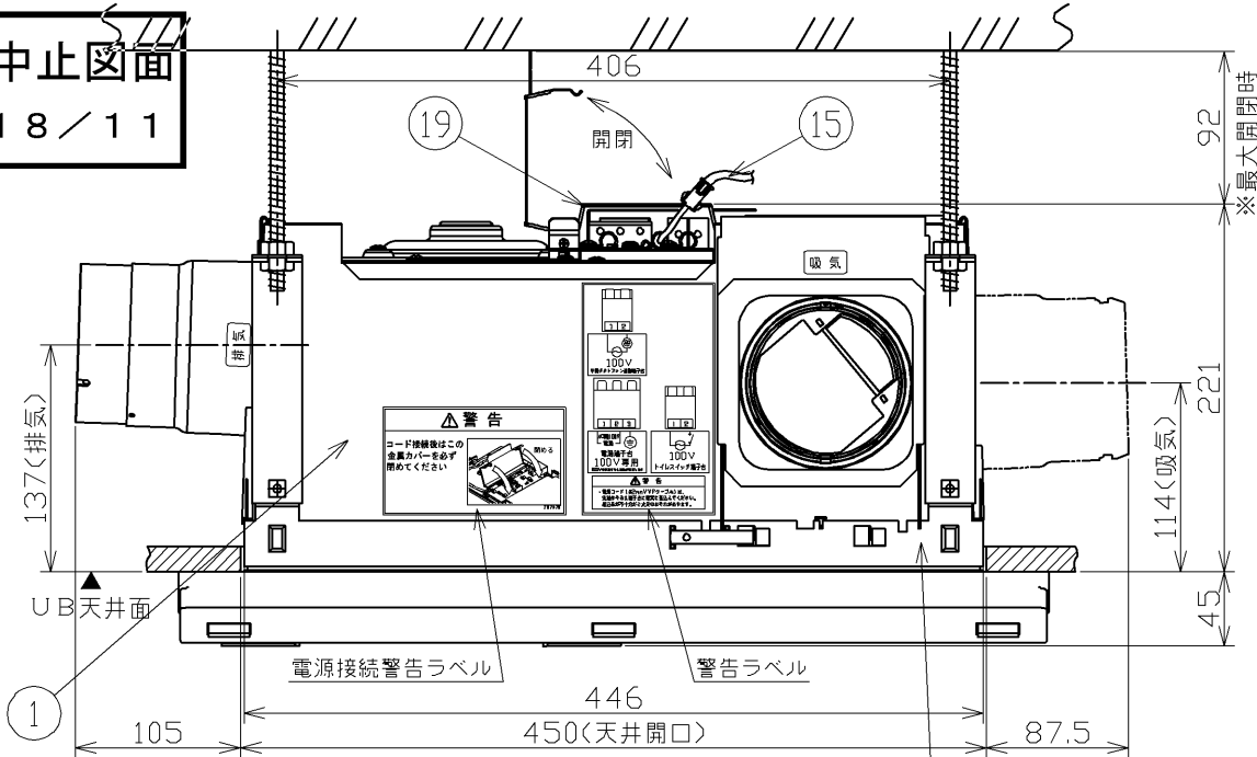
天井取付図 (1:5)
