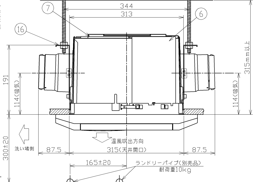
天井取付図 (1:5)
