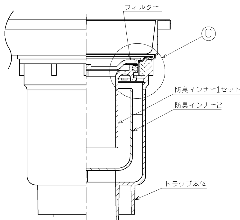
トラップ詳細図
