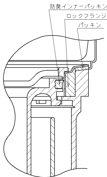
C部詳細図(1:1)
