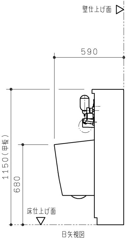
B矢視図
