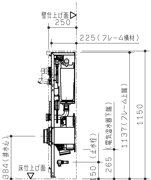
R 視図
