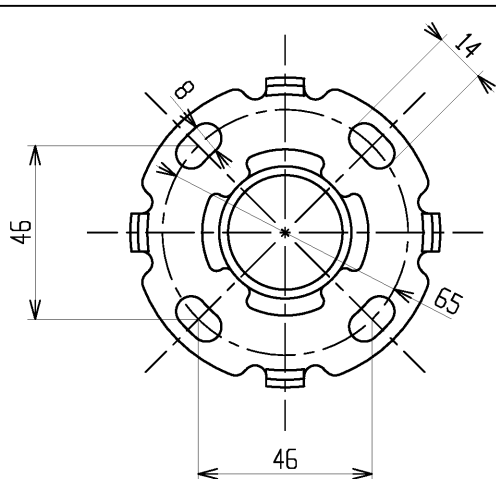
取付座詳細(1:2)
