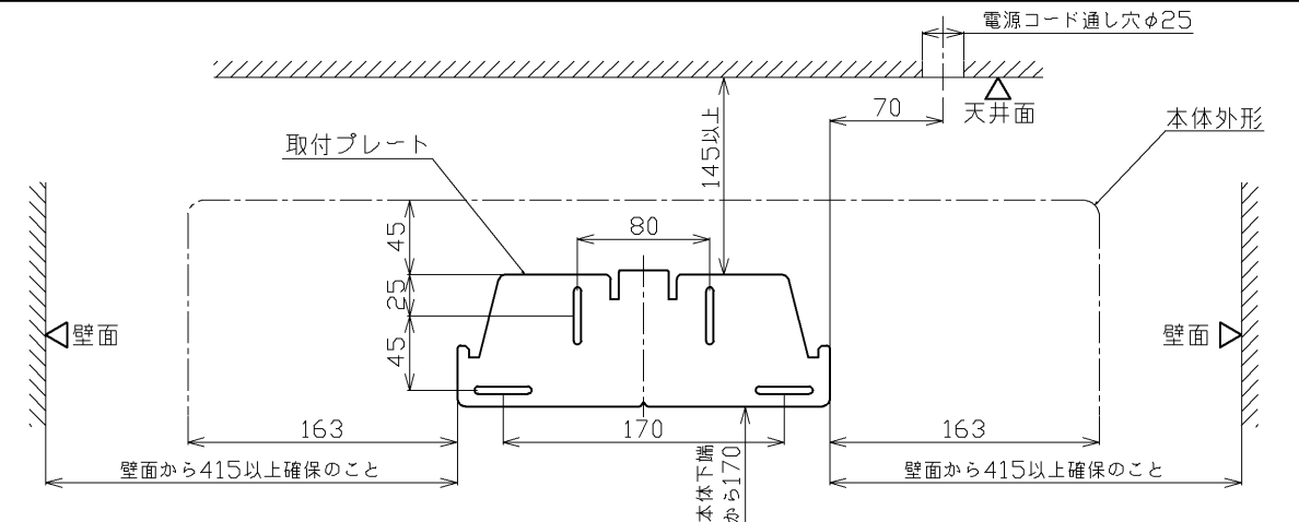
製品取付位置
