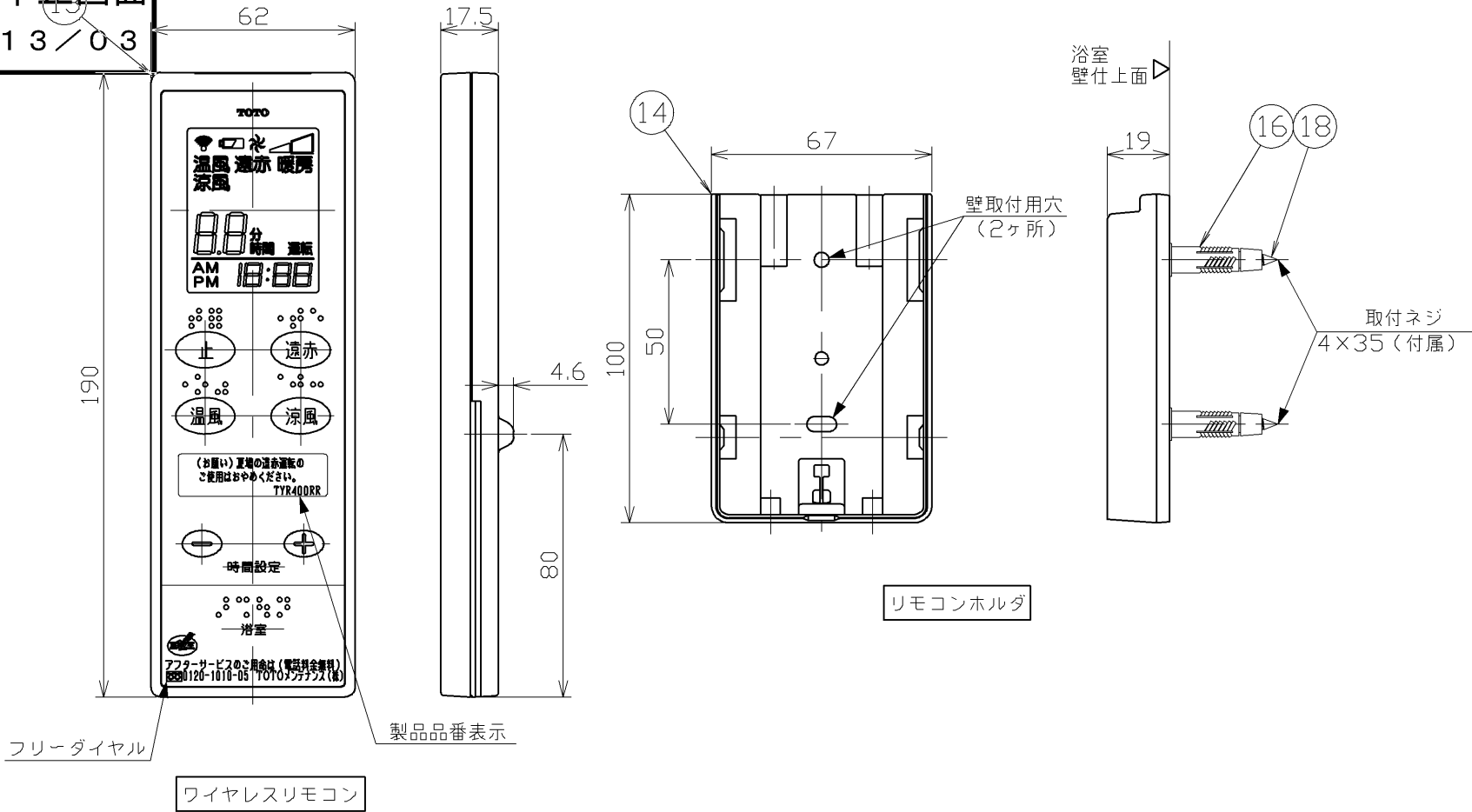
リモコン組品外観（１：２）
