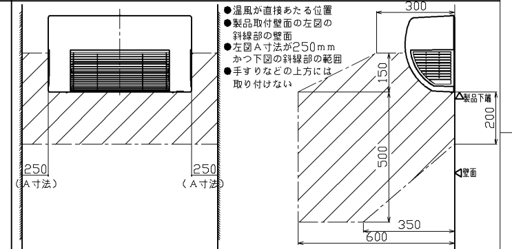
製品取付条件（下記の範囲内に、シャワーなどの器具がないこと）
