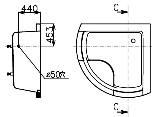
断面C-C
