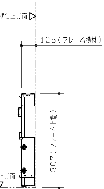
Q 視図
