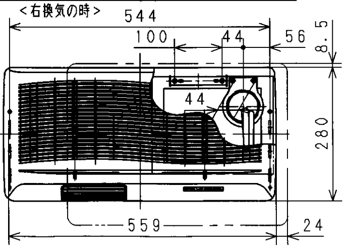
浴室ユニット（木枠内にダクトを通す場合）
