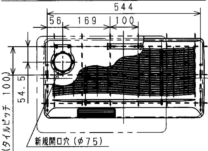
浴室ユニット（新規開口穴にダクトを通す場合）
