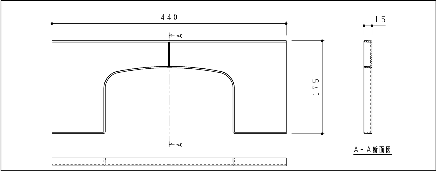
底板・間口大・奥行大（右）
