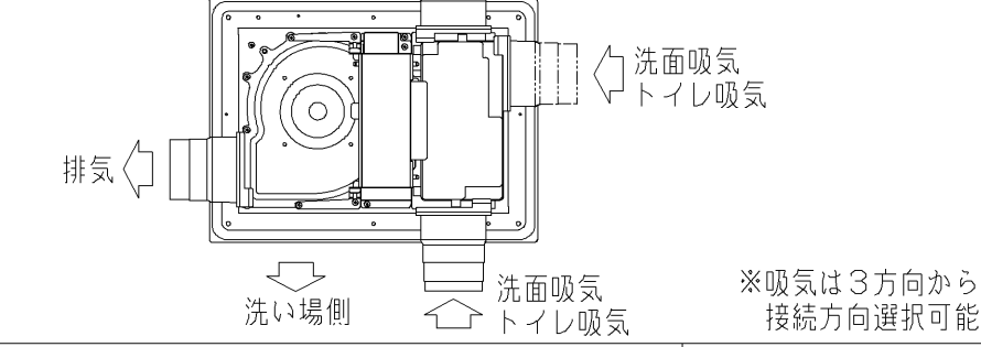
天井裏から見た図 <工場出荷時>
