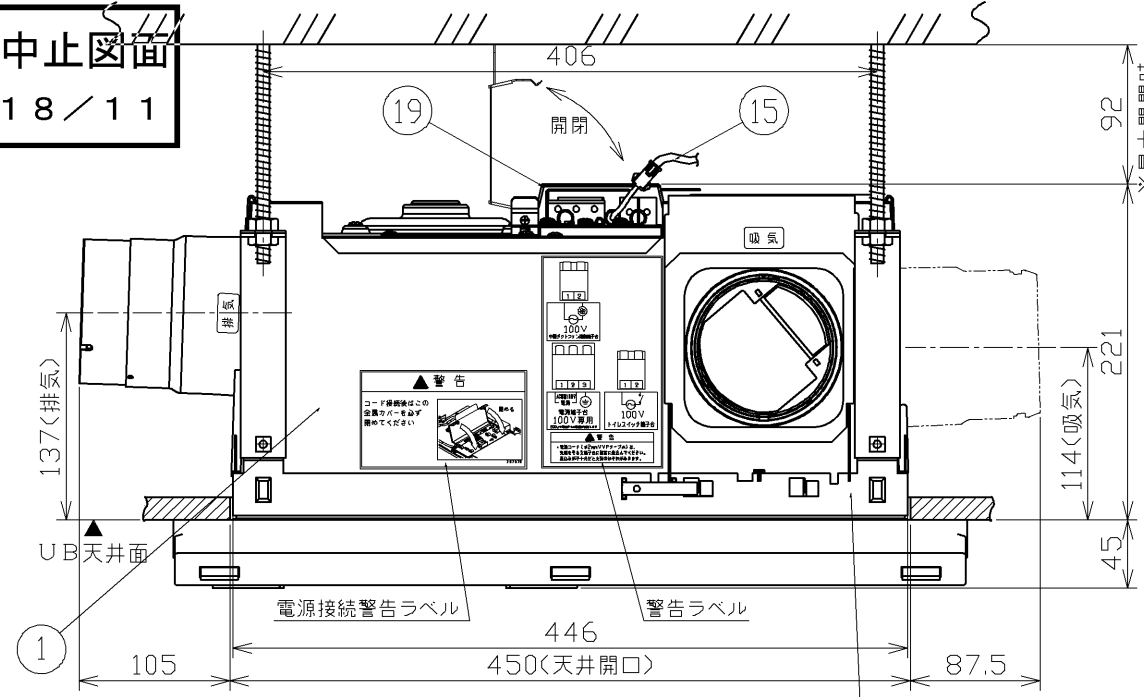
天井取付図 (1:5)
