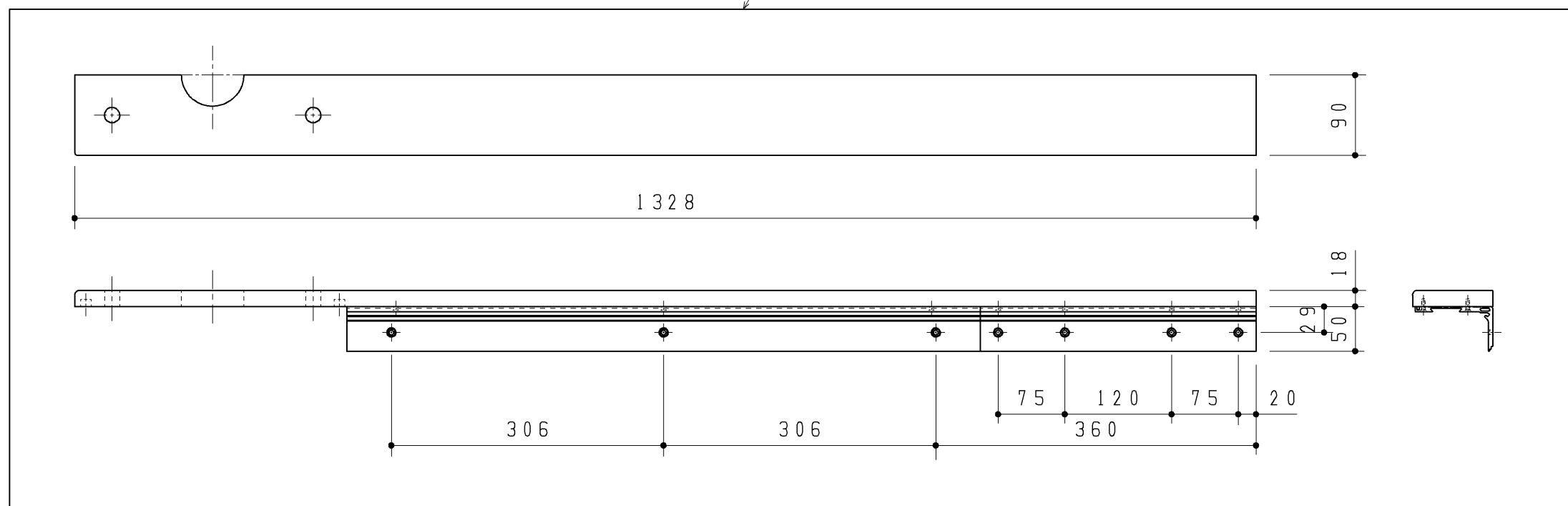
カウンター-L (埋込・1500 小)
