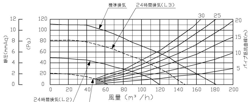
静圧風量特性曲線（換気運転時）
