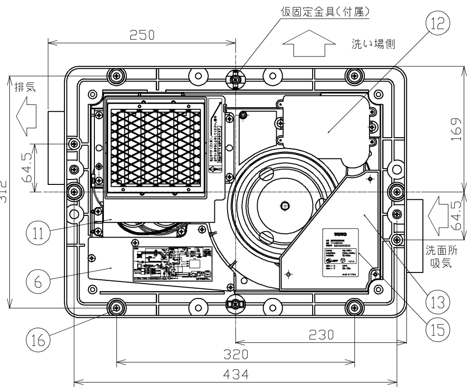
天井取付図 (1:5)
