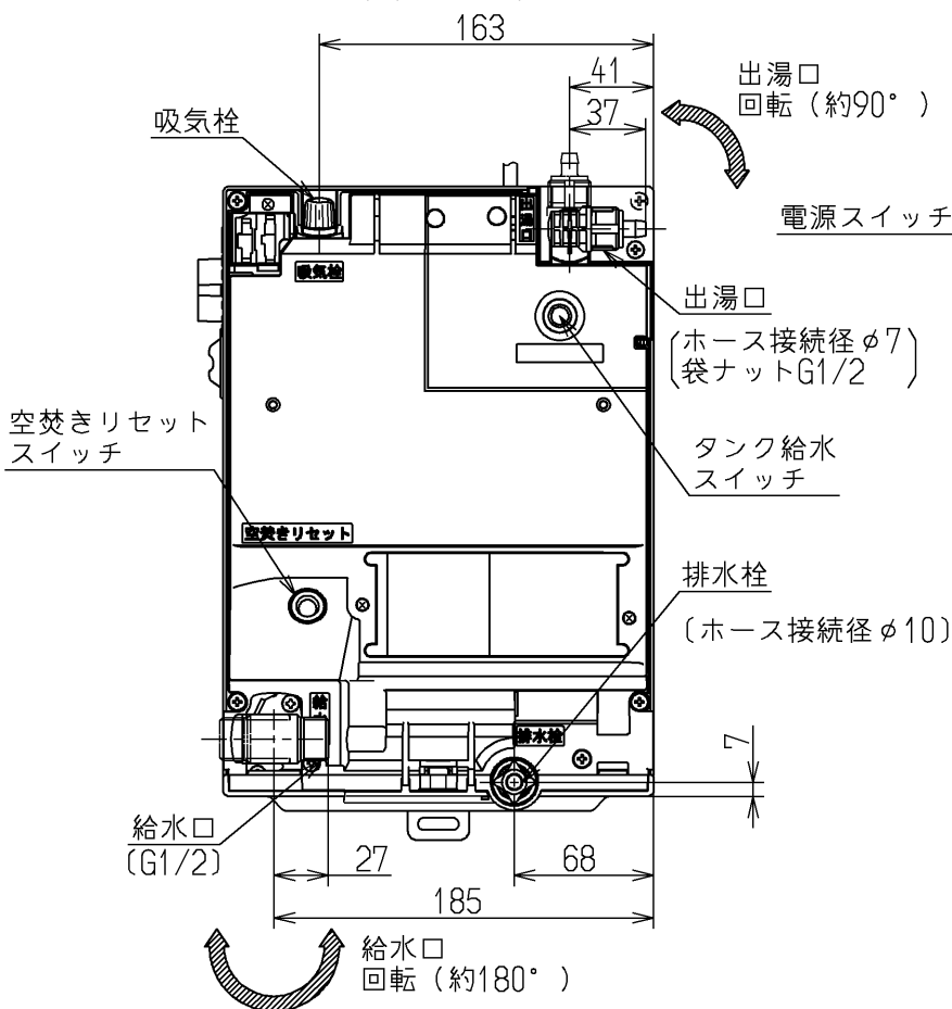
■化粧カバー取外図
