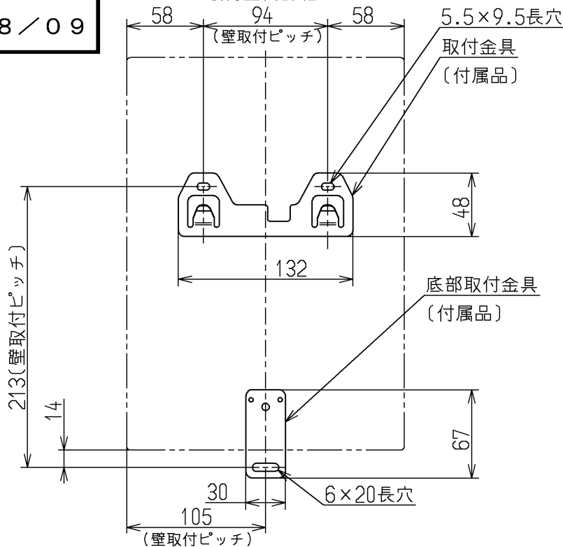
■取付金具詳細図
