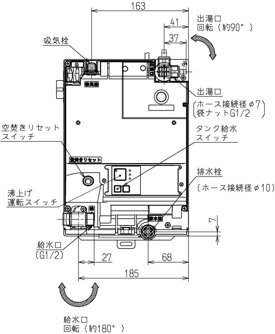
■化粧カバー取外図
