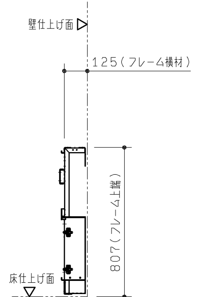
P 視図
