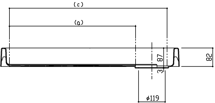
断面A-A
