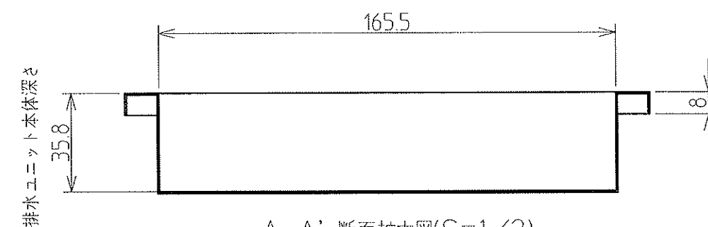
A-A' 断面拡大図(S=1/2)
