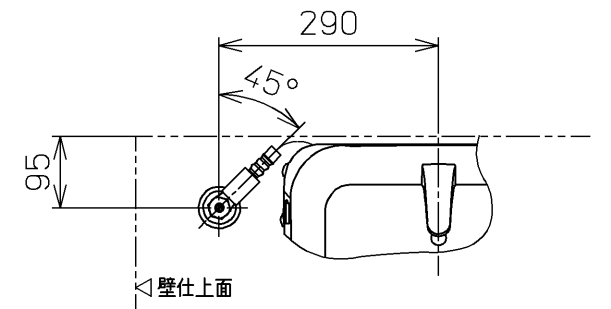
平面图
