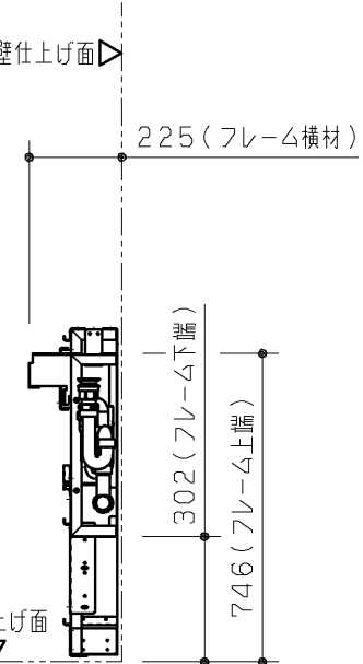
P 視図
