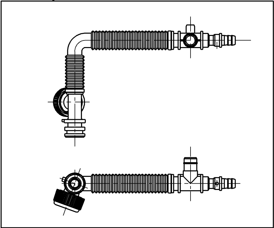
ボールタップ変更ユニット(8L用)
