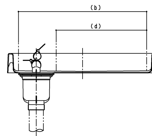
断面B-B
