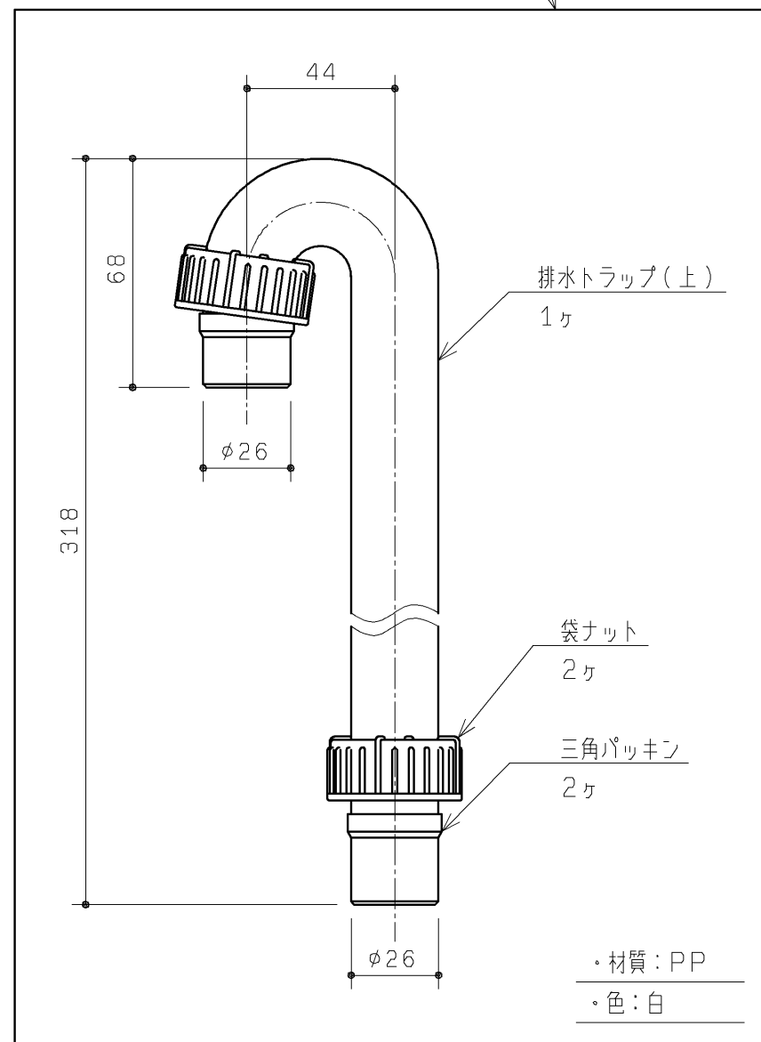
排水トラップ(上)セット(L=318) 1ヶ
