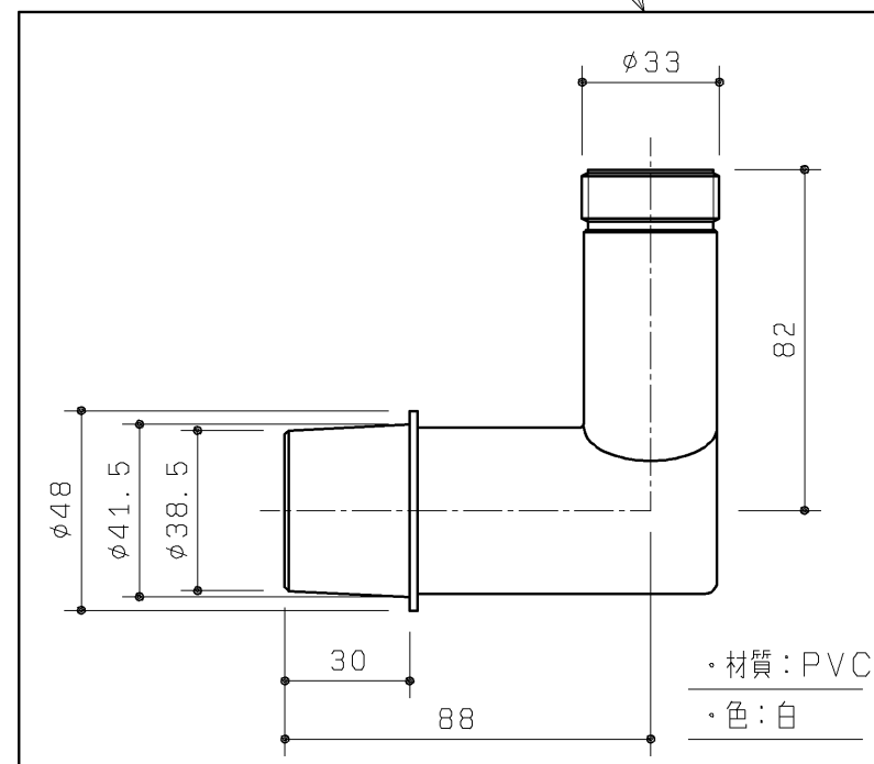
排水アダプター 1ヶ
