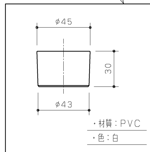
排水アダプター 1ヶ
