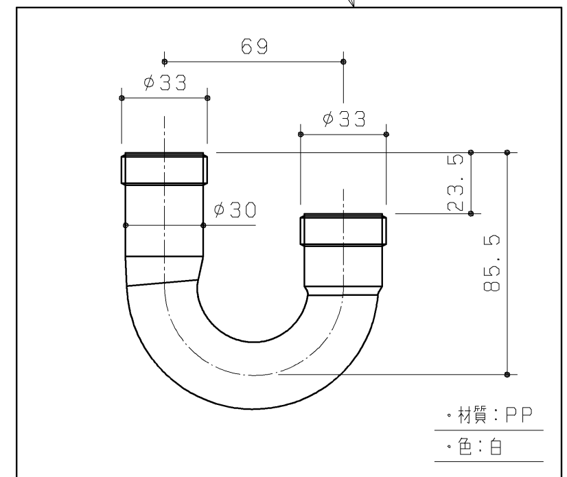
排水トラップ(下) 1ヶ
