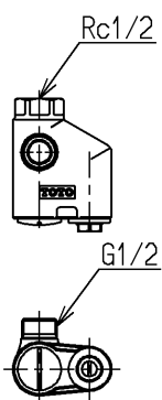
止水栓部(2ヶ入り)
