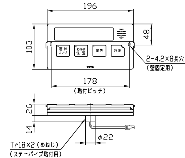
■ 浴室リモコン（別売品：RAC135F） ※ステーパイプ、カセットケースは浴室用屋外カバーセット（1：5） （別売品：RHA1360N）として準備。
