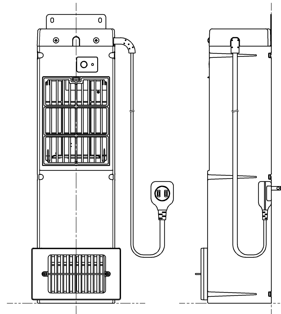
手洗器下キャビネットR勝手の場合(組立時)
