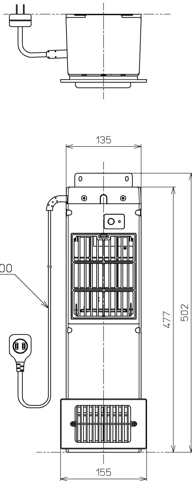
手洗器下キャビネットL勝手の場合(組立時)
