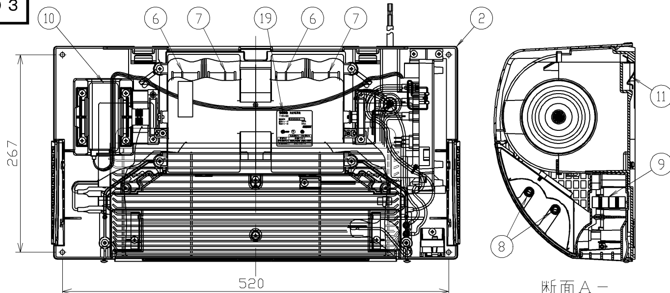
本体取付穴寸法（1：5）
