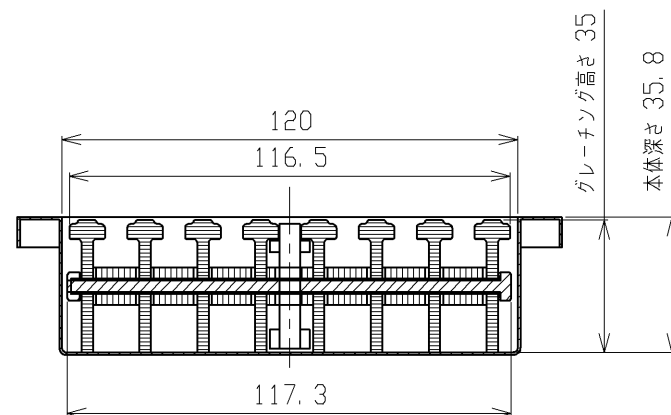
A-A断面詳細図 (1:2)
