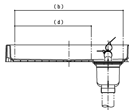
断面B-B
