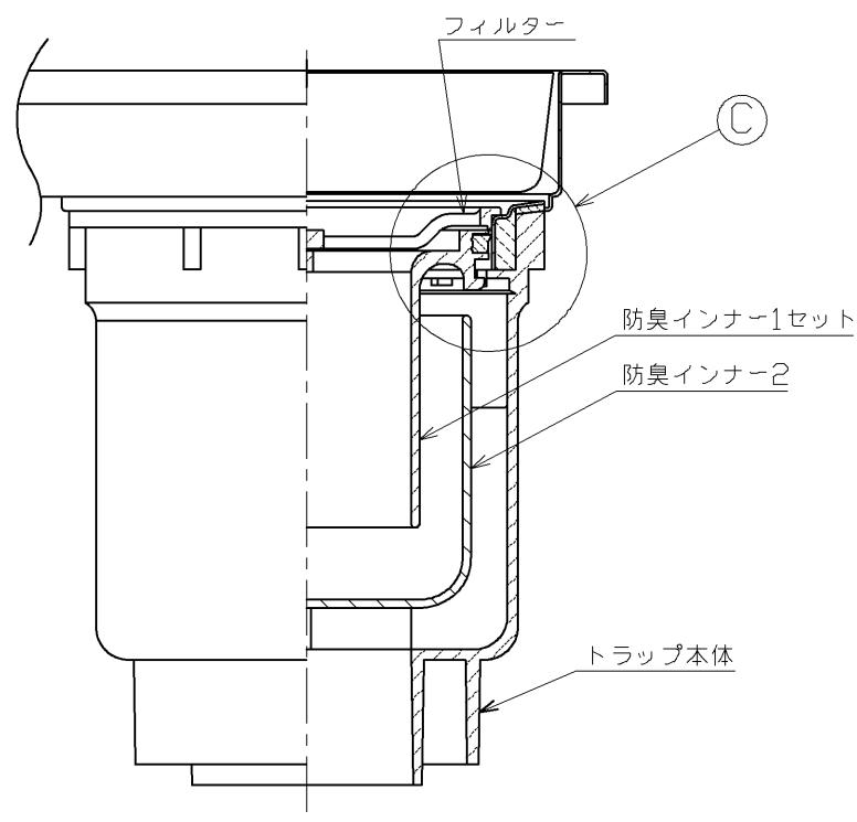
トラップ詳細図
