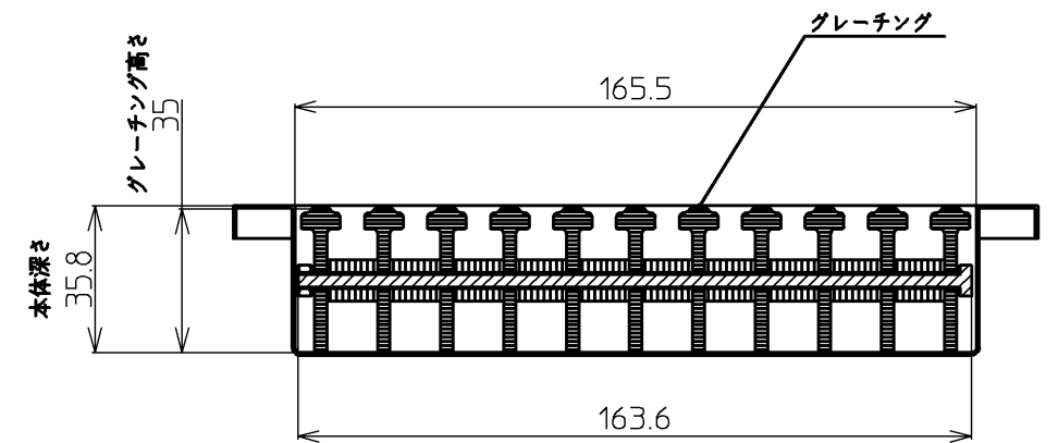
A-A' 断面拡大図(S=1/2)
