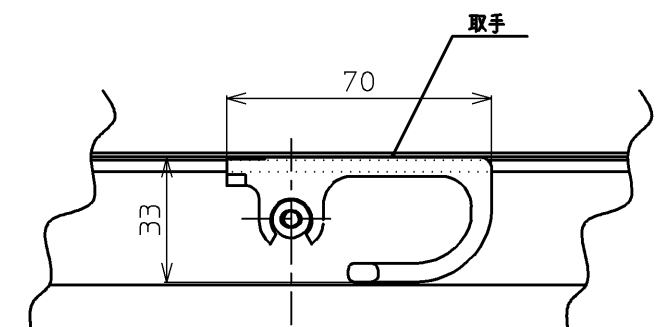
B-B' 断面拡大図(S=1/2)
