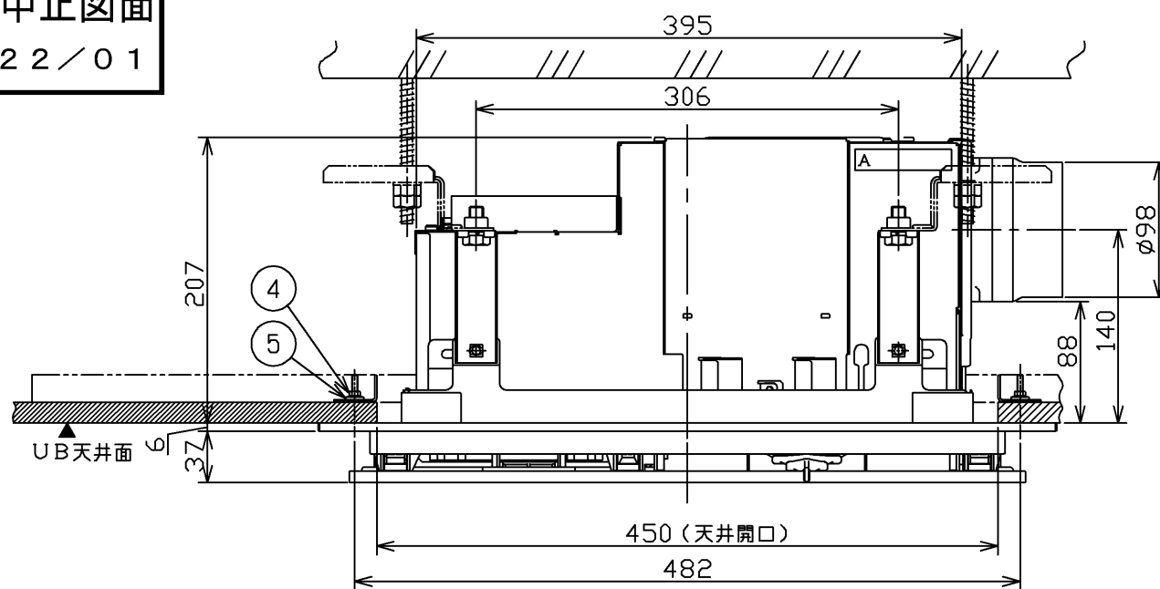
天井取付図
