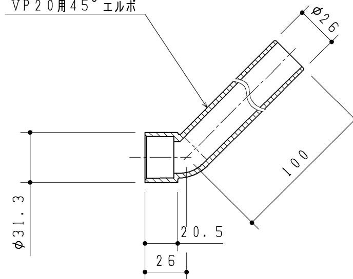
VP20用45°エルボ
