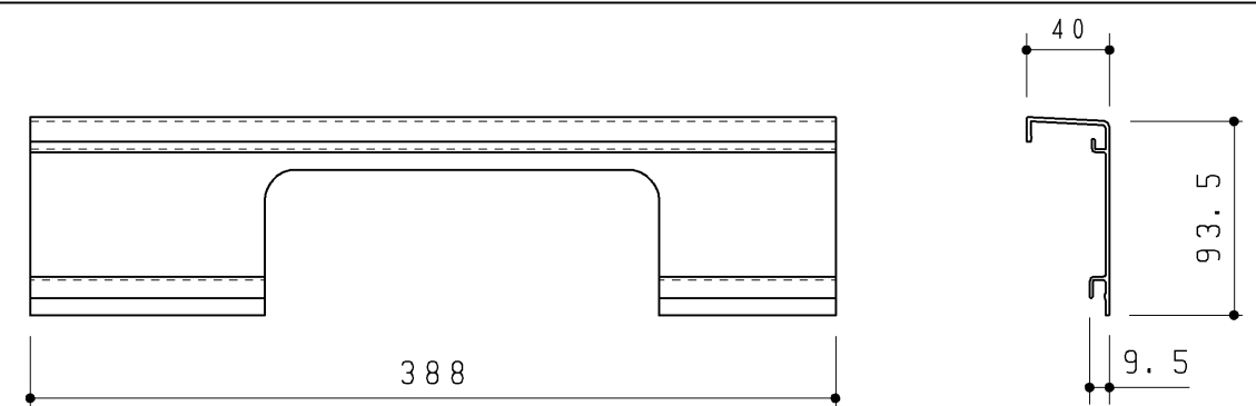
配管カバーR (間口小) (ホワイト)
