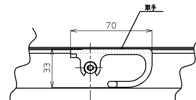
B-B' 断面拡大図(S=1/2)
